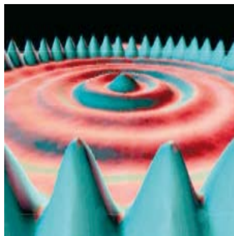
Mit der Spitze eines Tunnel-Mikroskops ringförmig angeordnete Xenon-Atome auf eine Kupfer-Oberfläche. Quelle: IBM
